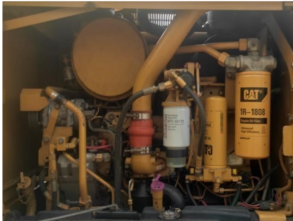
Fotografía No. 6 Vista Motor
